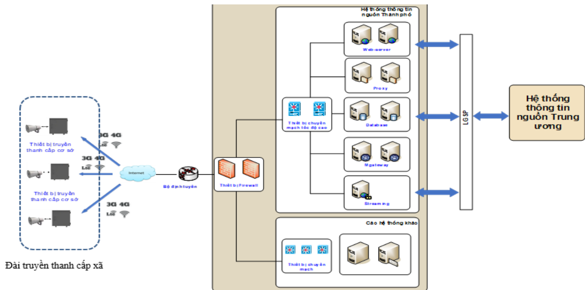
Mô hình tổng thể giải pháp Đài TTCS ứng dụng CNTT-VT
